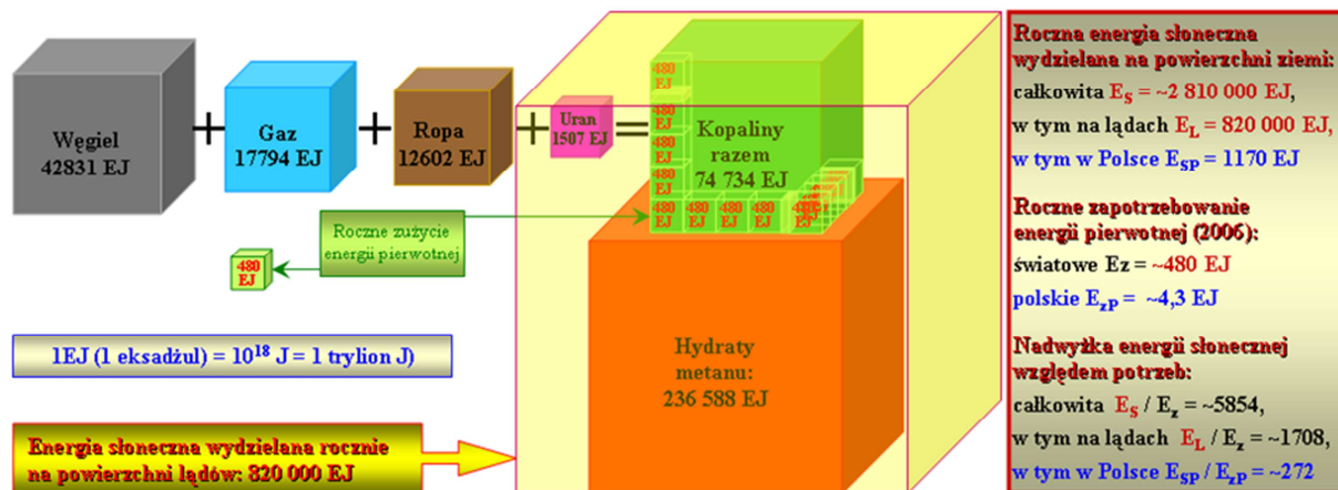
Rys. 16. Światowe zasoby energii pierwotnej [EJ] ze źródeł kopalnych, oszacowane z prawdopodobieństwem 95% wg danych za rok 2005 [10] i bilans energii słonecznej. Średnie przeliczniki wg World Energy Council [11].
