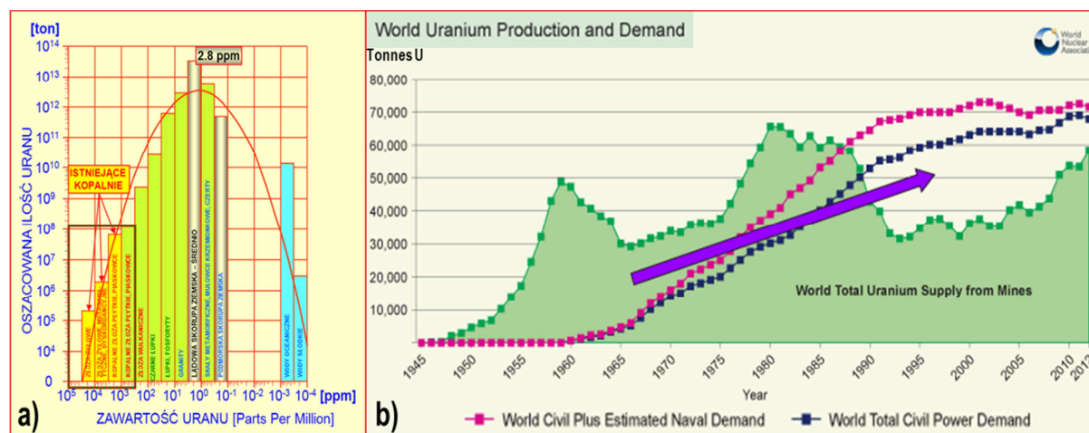
Rys. 11. Uran na ziemi: a) ilość i koncentracja uranu w różnych typach złóż lądowych i podmorskich oraz w wodach oceanicznych [43]; b) uran w latach 1945 ÷ 2012: światowe zapotrzebowanie: ■ - do celów cywilnych, ■ - całkowite (cywilne oraz dla marynarki); ■ - światowa produkcja roczna [44]. ➔ Deficyt (wg WNA) pokrywany był z pozostałych źródeł (malejące zapasy cywilne i zapasy wojskowe związane z redukcją broni jądrowej, pluton i uran z przerobu wypalonego paliwa 20 ).
