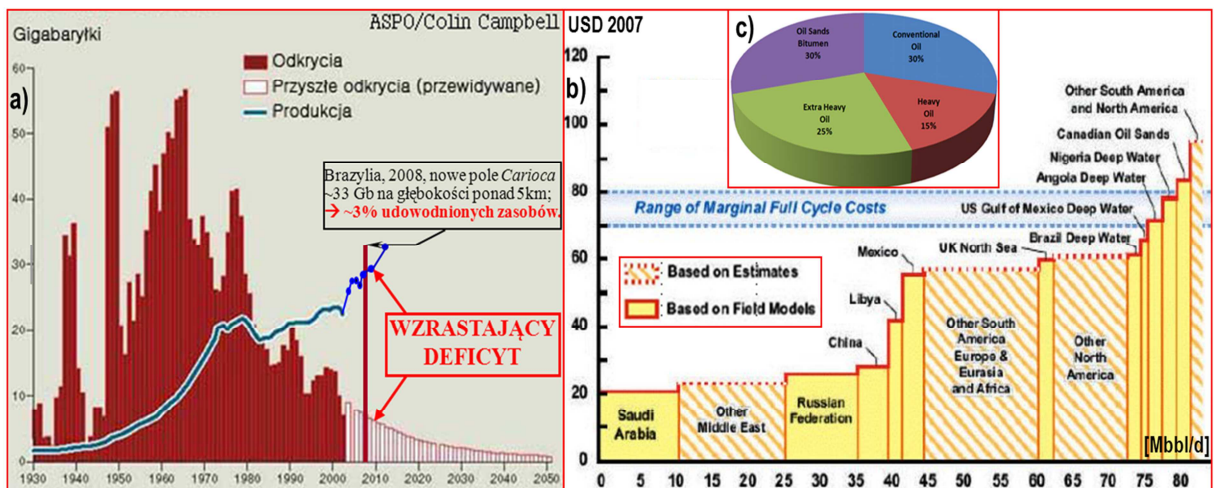
Rys. 5. Objawy kryzysu naftowego: a) wzrastający deficyt ropy naftowej [9], uzupełnienia własne wg [15] oraz o zasobności złoża Carioca wg [16] (niepotwierdzone); b) struktura kosztów ([USD], kurs wg 2007 r.) skumulowanego zużycia dziennego ([Mbb/d] – megabaryłek/dziennie) ropy naftowej różnego rodzaju, pochodzących z różnych złóż i z różnych źródeł [17]; c) struktura światowych zasobów czterech podstawowych odmian ropy naftowej: ■ - konwencjonalnej, ■ - ciężkiej, ■ - superciężkiej, ■ - z łupków i piasków bitumicznych. Mnożniki UE/PL: M – 10 6 (mega, milion); G – 10 9 (giga, miliard).
