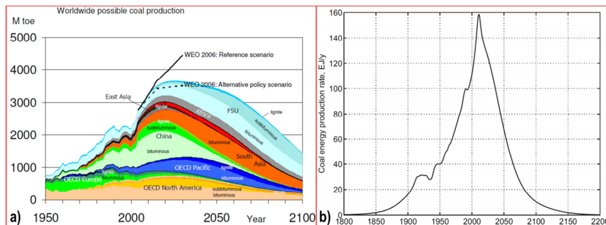
Rys. 10. Węgiel na świecie: a) historia i prognozowane scenariusze produkcji węgla (w [Mtoe]) 18 w latach 1950 ÷ 2100; b) model peak coal (wg teorii Hubberta), obejmujący produkcję (w [EJ/r]) wszystkich rodzajów węgla na całym świecie w latach 1800 ÷ 2200 [39].
